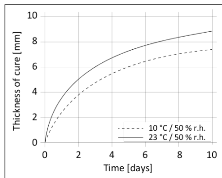
Diagramma 1: velocità di indurimento per Sikaflex®-292i
